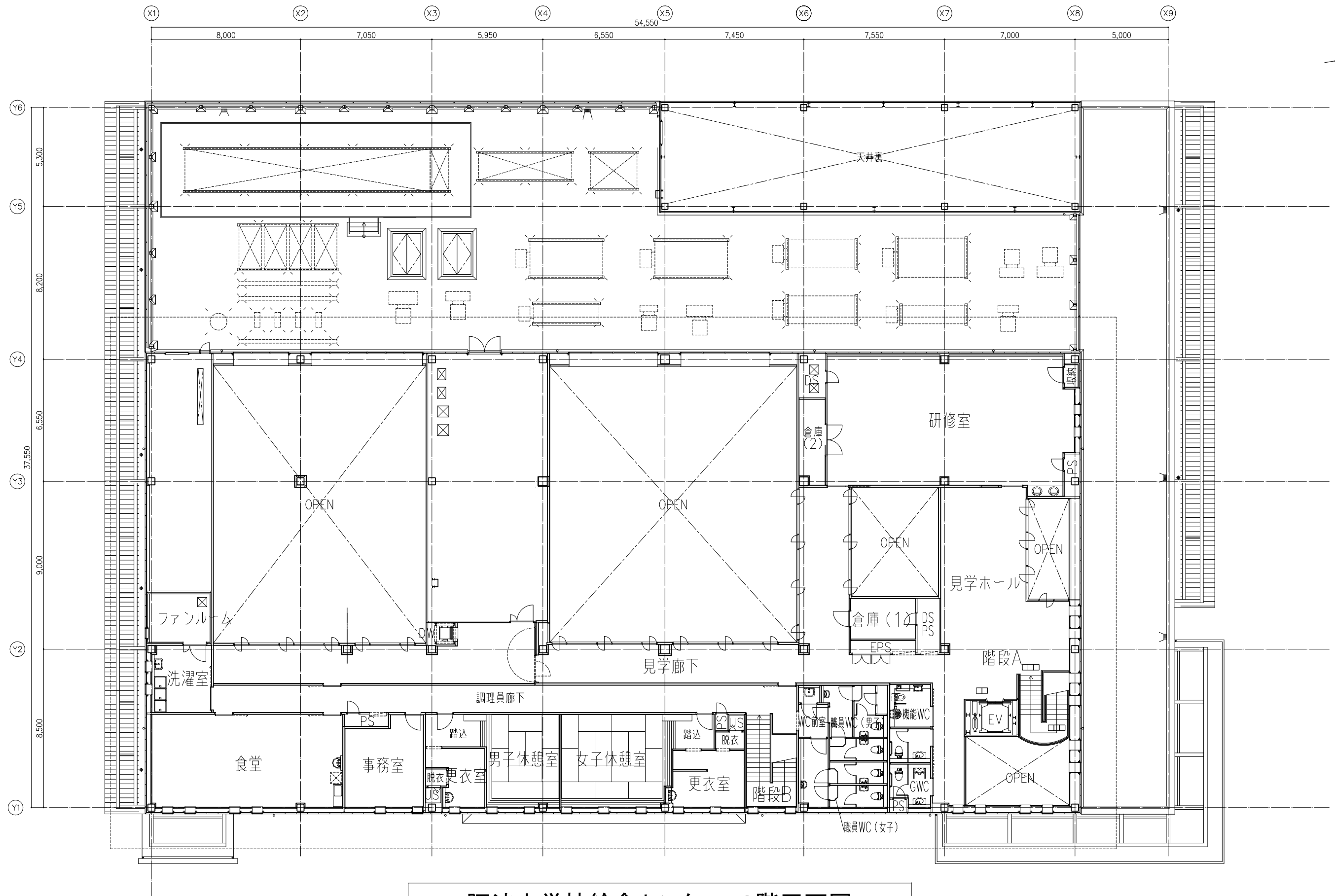
阿波市学校給食センター 2階平面図
