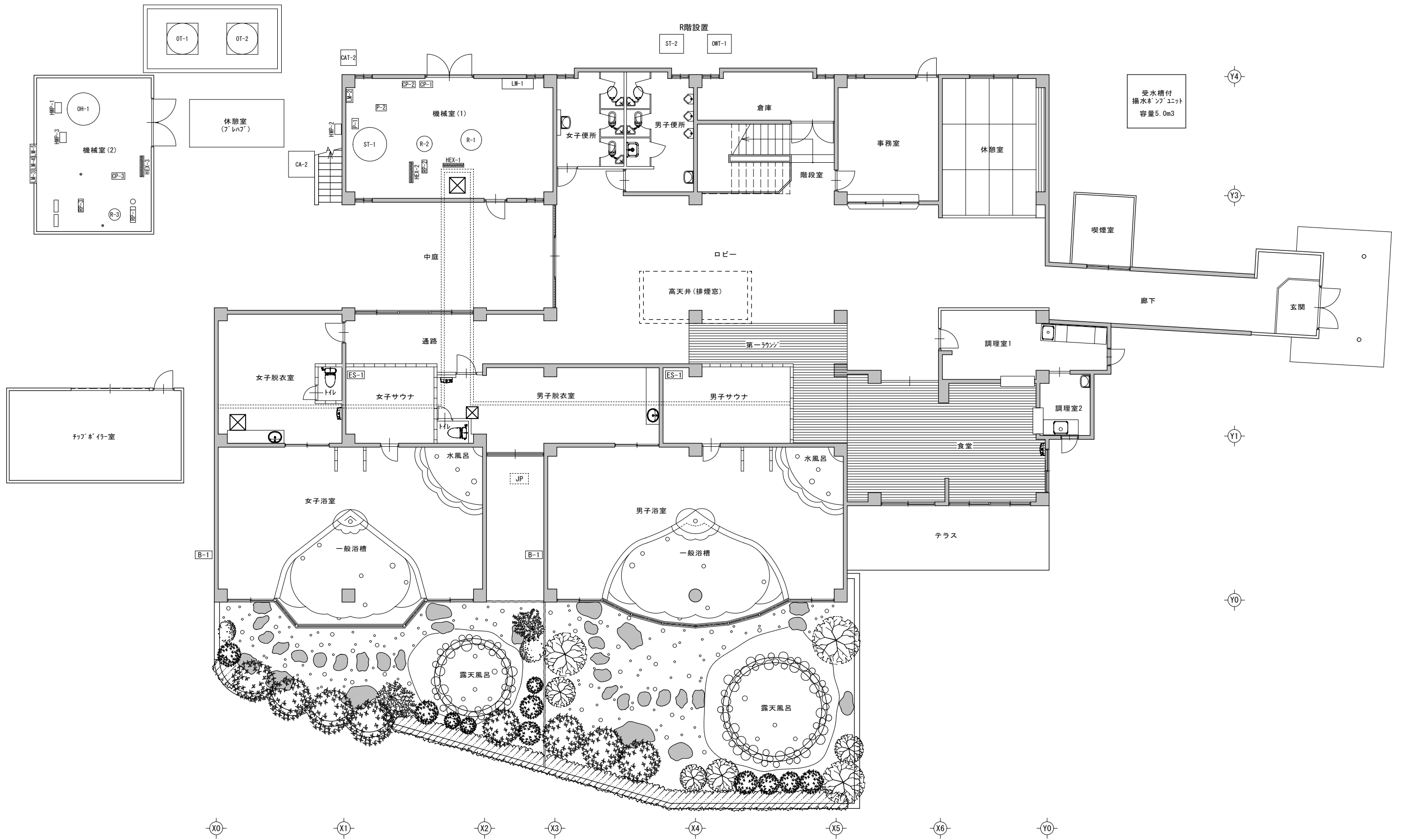
現況 1階平面図
