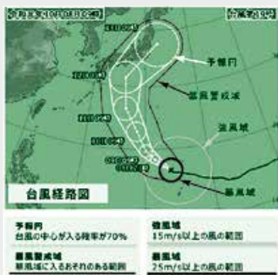
図2 台風経路予測
