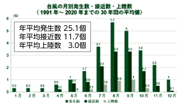
図1 台風の月別発生数・接近数・上陸数
