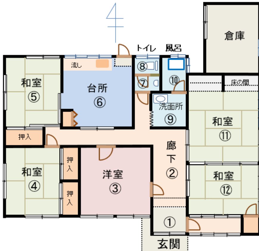
間取内訳
