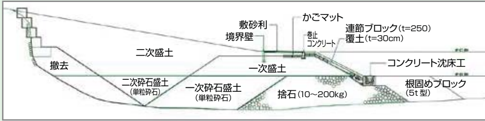
図 標準断面図
