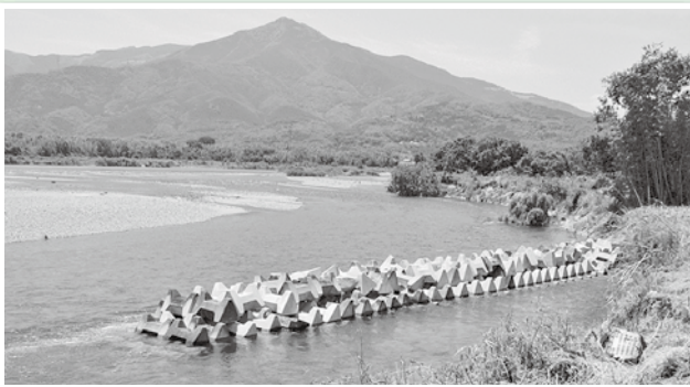
水制工の設置状況
